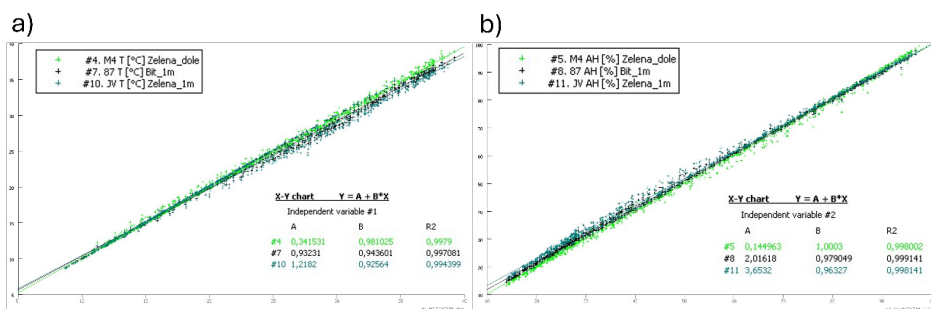
Obr. 7 Lineárna regresia a) teploty vzduchu a b) vlhkosti vzduchu pre rôzne povrchy strechy a výšky meraní nad povrchom); bit = bitumenová strecha, Zelena = zelená strecha, dole = meranie tesne pri povrchu strechy, 1m = meranie v 1 metri nad povrchom
