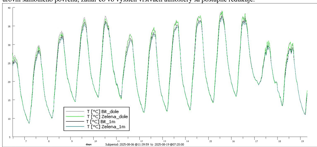
Obr. 5 Priebeh teploty vzduchu (°C) počas vybraných horúcich letných dní (6.–19.8.2025); bit = bitúmenová strecha, Zelena = zelená strecha, dole = meranie tesne pri povrchu strechy, 1m = meranie v 1 metri nad povrchom
