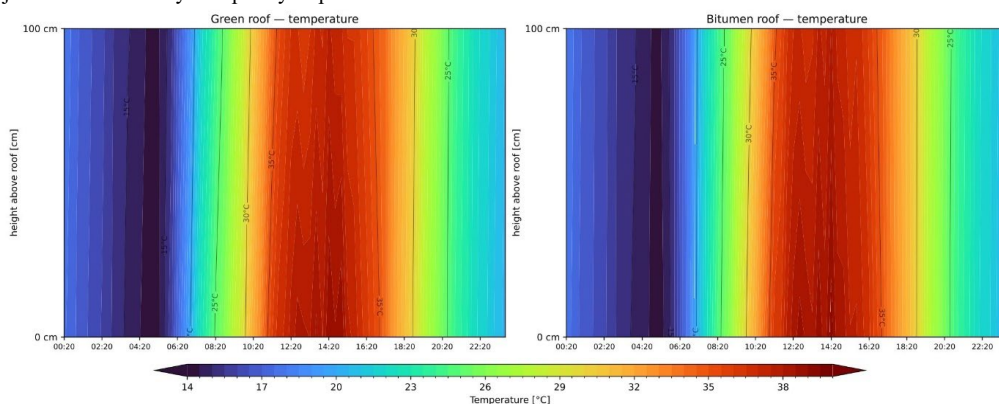
Obr. 10 Termoizoplety zo dňa 15.8.2025
