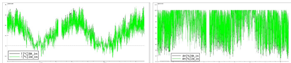
Obr. 9 Priebiež teploty vzduchu (°C, vľavo) a vlhkosti vzduchu (% , vpravo) vo výške 1 m nad povrchom strechy počas celého obdobia merania (29. 6. 2023 – 19. 8. 2025); Bit_1m = bitúmenová strecha, Zel_1m = zelená strecha
