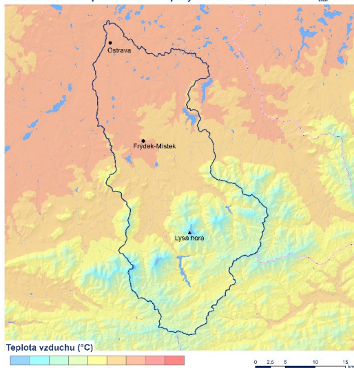
Ostravice – normál průměrné roční teploty vzduchu 1991–2020
