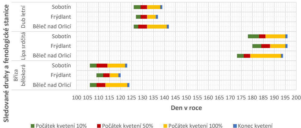
Graf 4: Časová osa nástupu průměrného trvání doby kvetení v letech 1991-2024 (Běleč nad Orlicí, Sobotín) a 1997-2023/2024 (Frýdlant)
