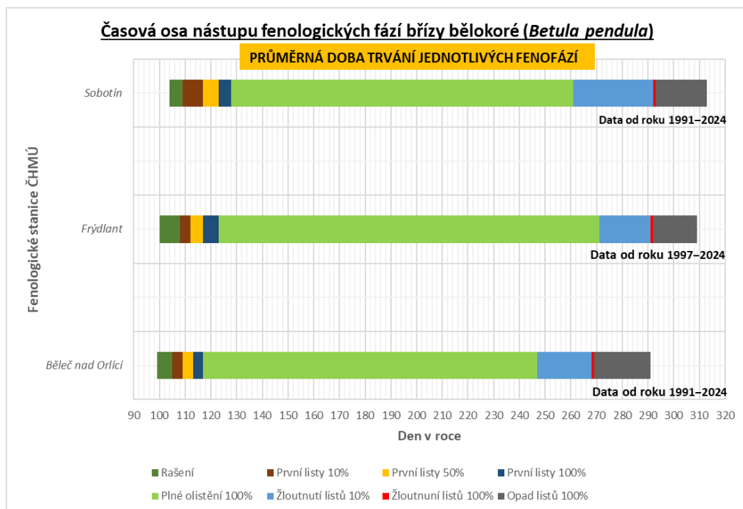
Graf 1: Časová osa nástupu fenologických fází břízy bělokoré ( Betula pendula ) v období 1991–2024 (Běleč nad Orlicí, Sobotín) a 1997–2024 (Frýdlant)
