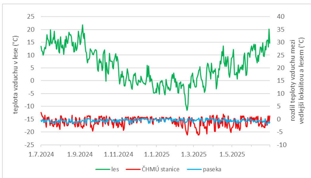
Obr. 3 Minimální denní teploty vzduchu v lese a rozdíly mezi ČHMÚ stanicí a lesem a pasekou a lesem Fig. 3 Minimum daily air temperatures in the forest and differences between the ČHMÚ station and the forest and the clearing and the forest
