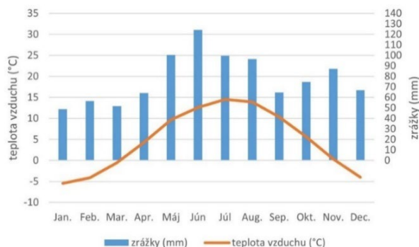
Obr. 2 Klimadiagram výskumnej lokality
