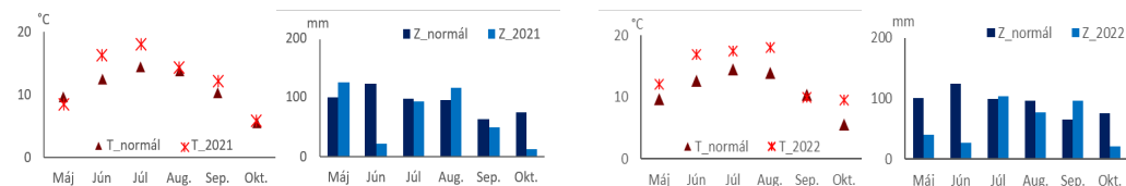
Obr. 3. Priemerná mesačná teplota vzduchu a úhrny zrážok za rok 2021 (vľavo) a 2022 (vpravo) v porovnaní normálmi
