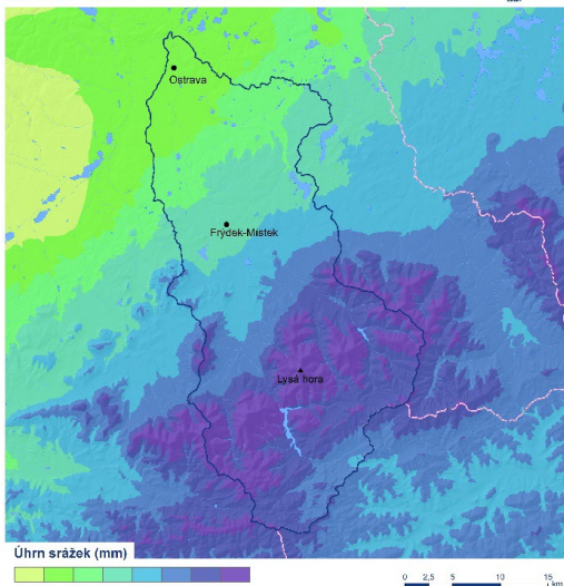
Ostravice – normál ročního úhrnu srážek 1991–2020
