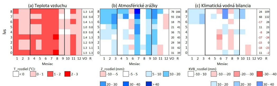
Obr. 3. Zmeny (a) teploty vzduchu, (b) atmosférických zrážok a (c) klimatickej vodnej bilancie v jednotlivých mesiacoch, vo vegetačnom období (VO) a v rámci roka (R) medzi klimatickými normálovými obdobiami 1961–1990 a 1991–2020
